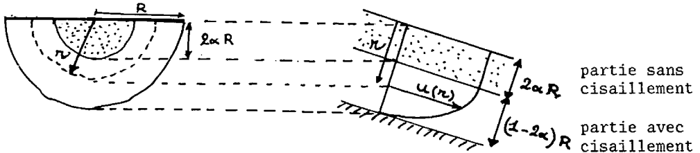
Figure 9.2 : Ecoulement laminaire de Bingham dans un demi-cercle
